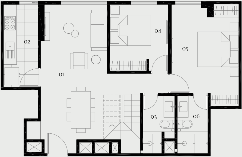
PRIMER NIVEL
