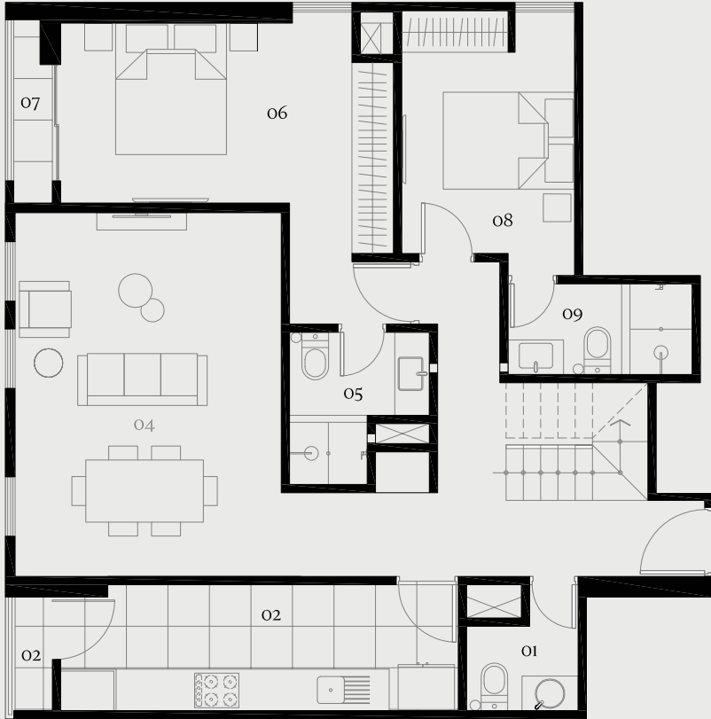
PRIMER NIVEL
