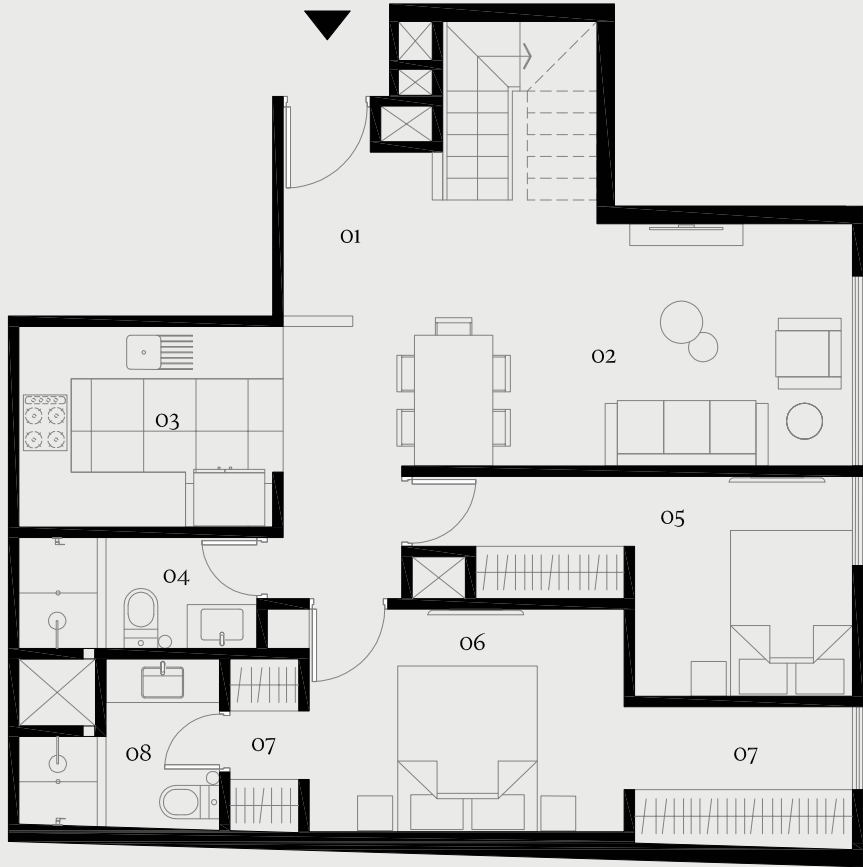
PRIMER NIVEL
